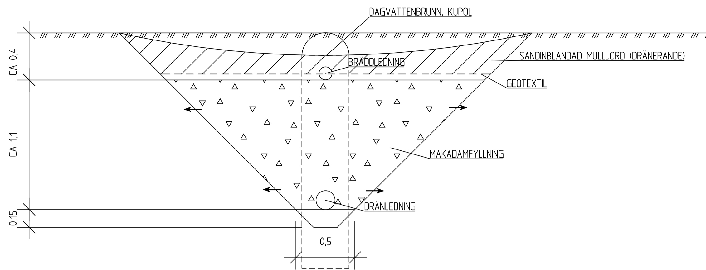
SEKTION A
