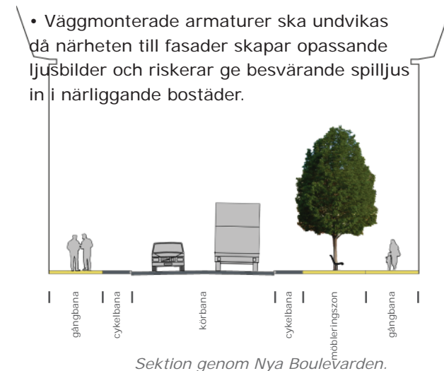
Sektion genom Nya Boulevarden.
