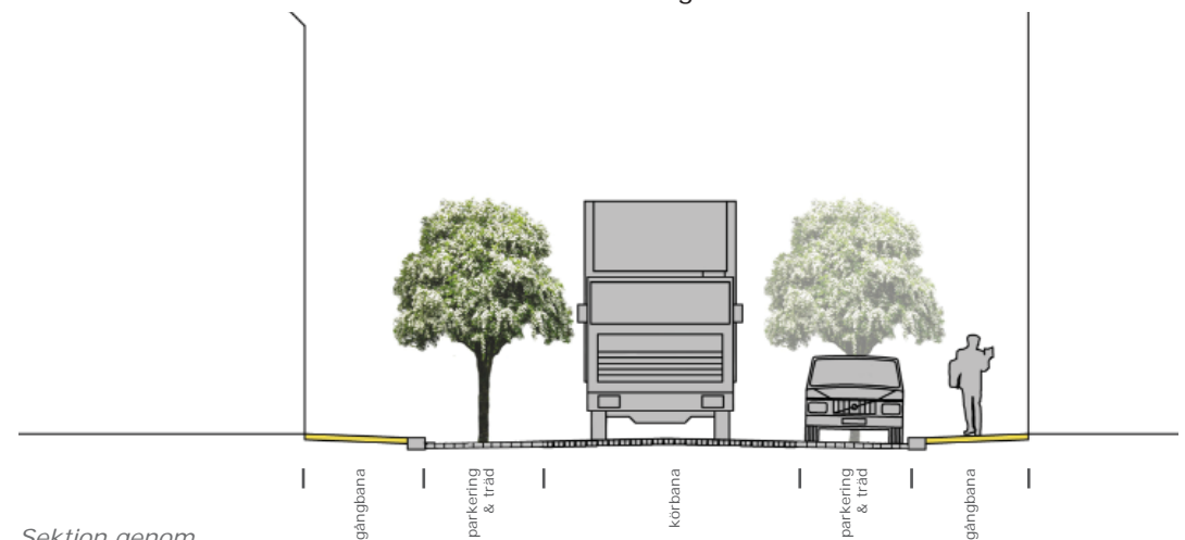
Sektion genom vallgata.
