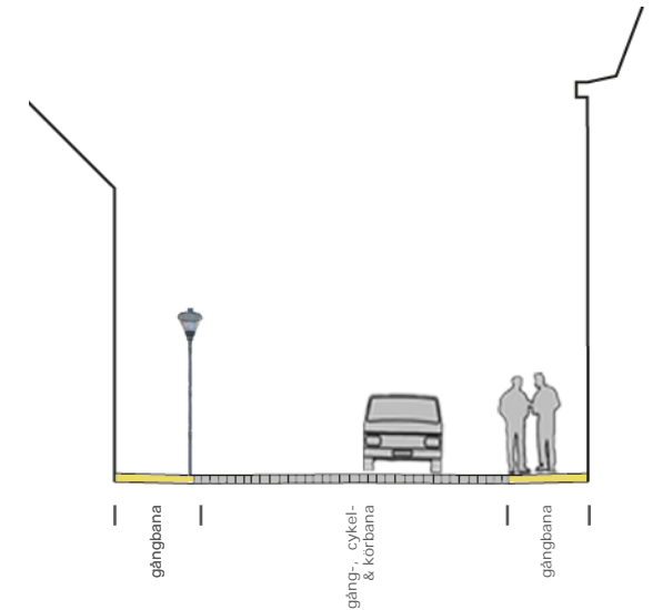
Sektion genom tvärgata med gång-, cykel- och biltrafik.
