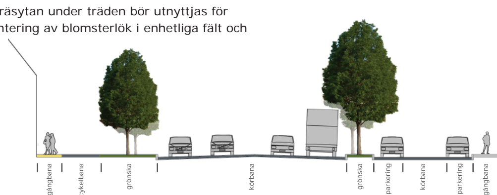
Sektion genom Södra Boulevarden.
