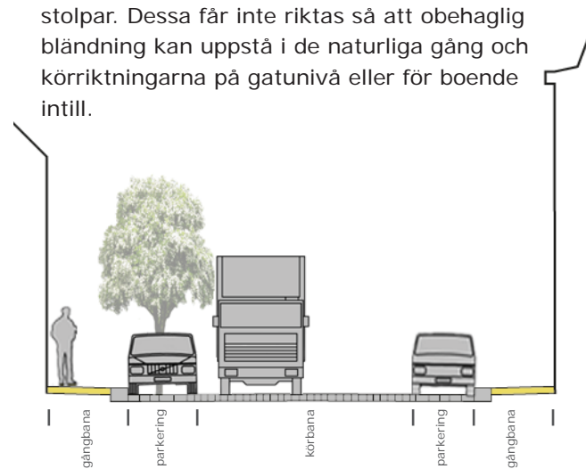
Sektion genom tvärgata med biltrafik.
