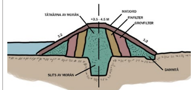
Skyddsvallen kan se ut som en jordhög, men är en komplicerad och kostsam konstruktion. Det fullständiga vallskyddet beräknas kosta över 1,5 miljarder kronor.
