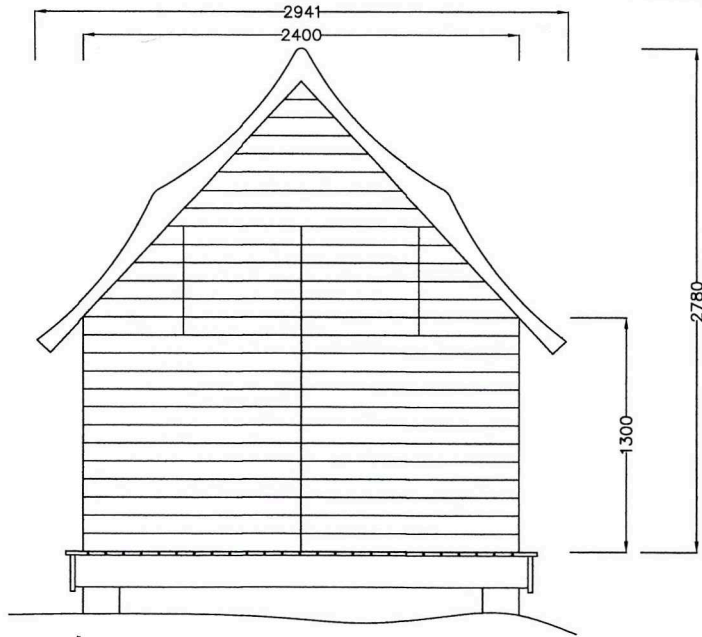
Fasad - Öst
