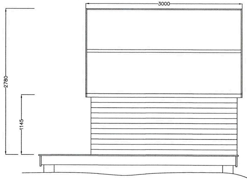
Fasad - Norr
