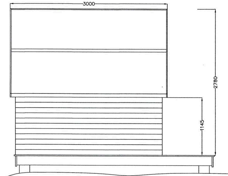
Fasad - Söder
