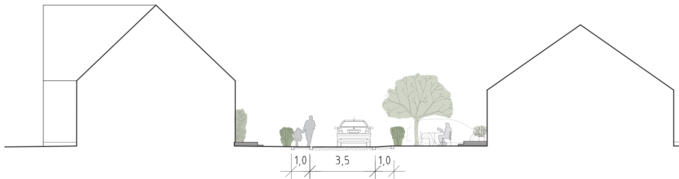
Sektion B-B genom sidogata
