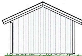
FASAD MOT VÄSTER
