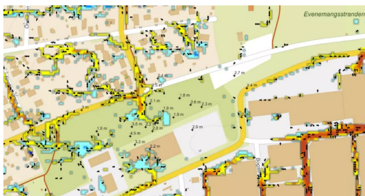
Skyfallsmodulering vid 100-årsregn för nuvarande
